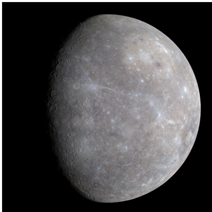
Abbildung 20 - Merkur
