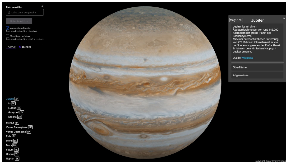
Abbildung 13 - App Screenshot
