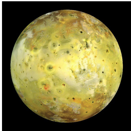
Abbildung 31 - Io (Jupitermond)
